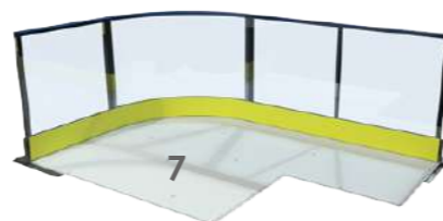
Boulonnage des rambarde entre-elles
