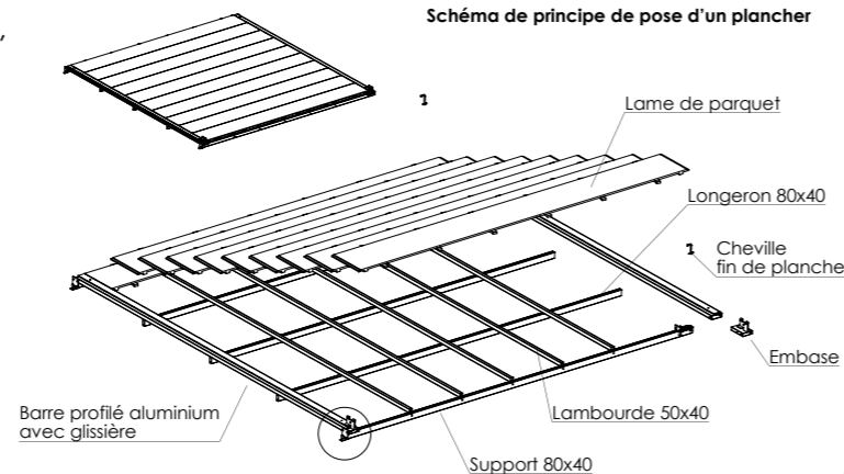
Schéma de principe de pose d'un plancher
