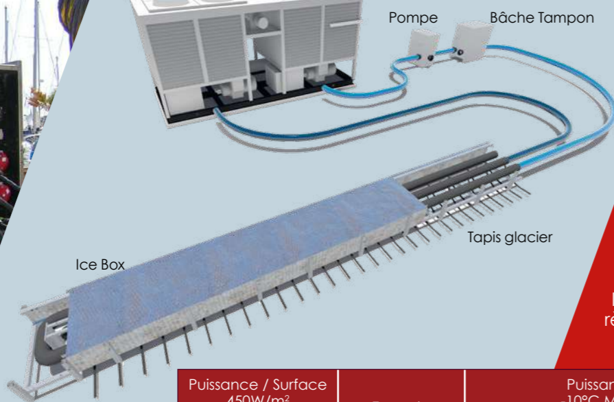
Groupe froid
